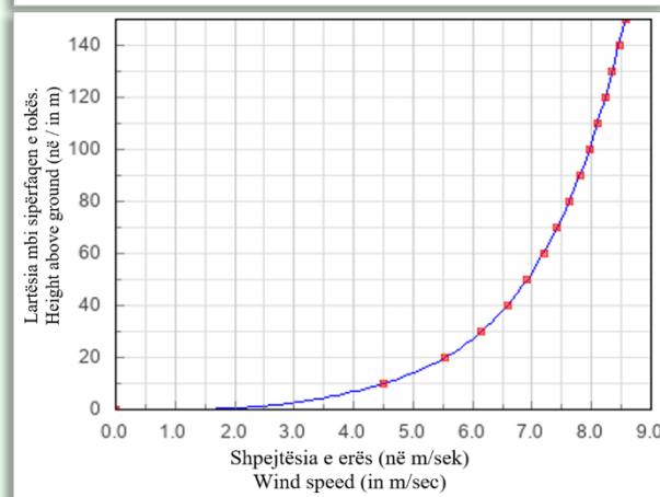
Figure Nr.44 Profili vertikal i shpejtësisë së erës. Vertical profile of wind speed.
